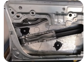
แผ่นซับเสียงหรือแผ่นลดการสั่นสะเทือนของคลื่นอัลตราโซนิก Ultrasonic Radar Damping Plate
